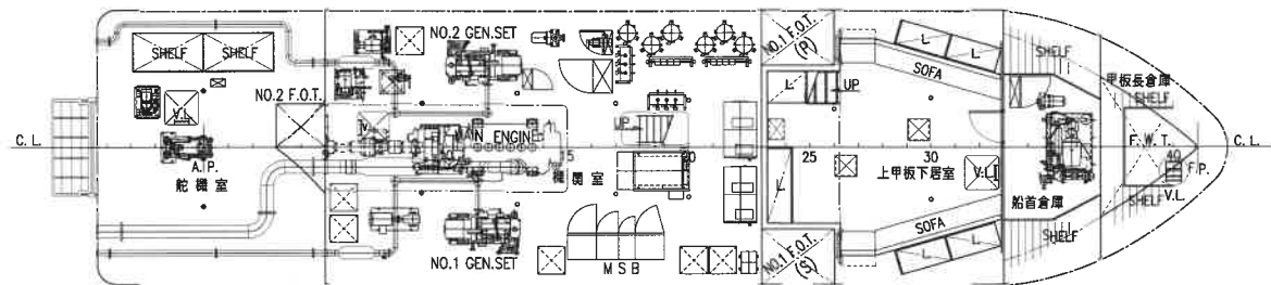
上甲板下平面
