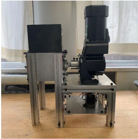
粉碎機
