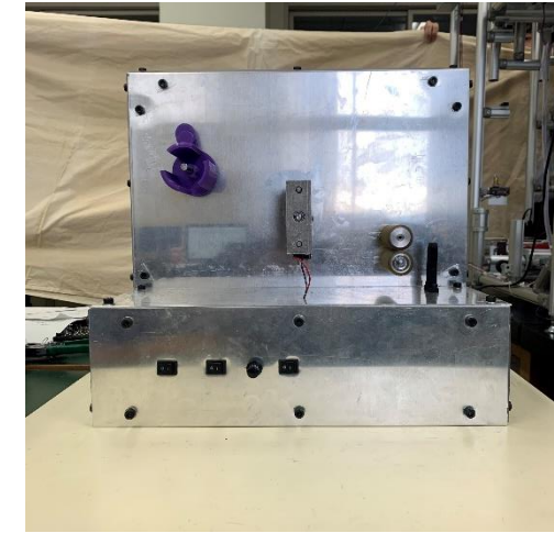
巻取機
