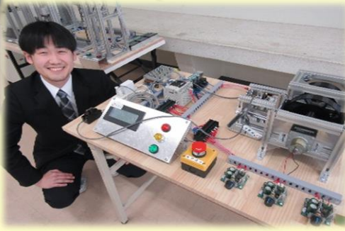
ねじ部品の自動計数及び排出 装置の製作
