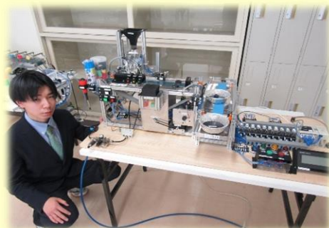
個数指定による部品の自動 供給装置の製作
