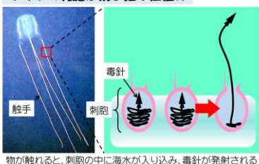
クラゲの刺胞が飛び出す仕組み
